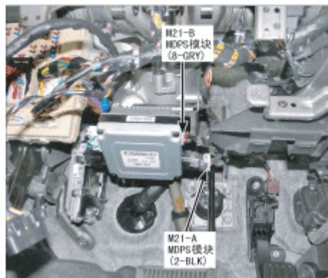
61. 转向柱
