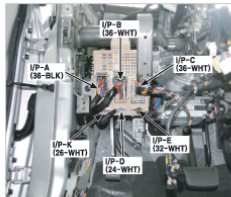
63. 仪表板左侧
